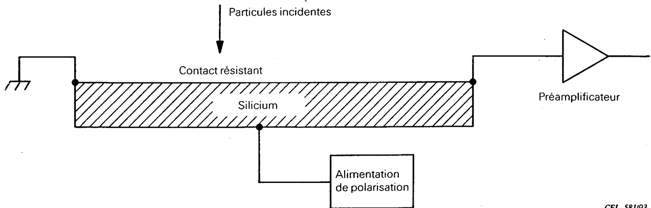
Figure 5 – Détecteur à localisation d'impact
