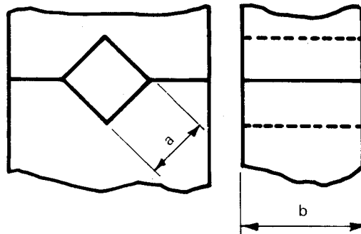
FIG. 3. — Dimensions des mâchoires pour sertissage carré (voir notes sous le tableau II — note 5 non applicable). Square crimp die dimensions (for notes, see below Table II — Note 5 not applicable).
