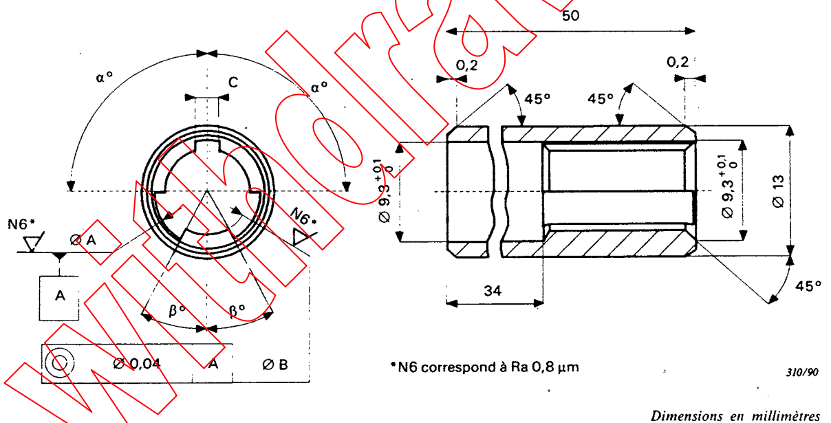
Figure 3 — Cotes des calibres d'interface des fiches (voir également tableau 3)
