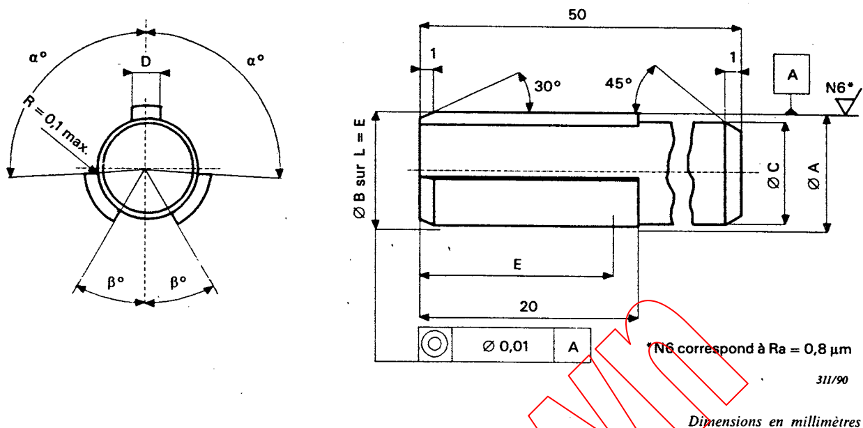
Figure 4 — Cotes des calibres d'interface des raccords (voir également tableau 4)
