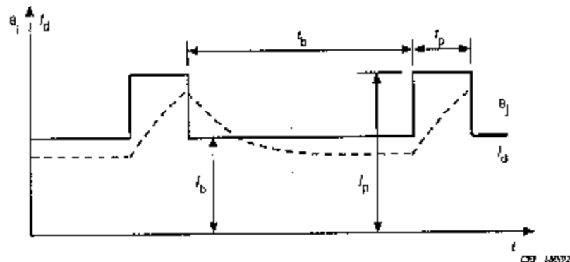
Figure 6 – Diagramme typique courant-temps pour régime de charge intermittente
