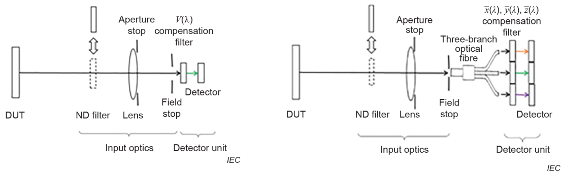
a) Luminance meter
