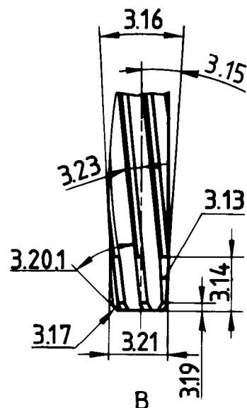
Entering end of hand reamer Extrémité avant de l'alésoir à main
