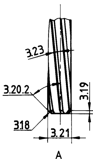
Entering end of parallel machine reamer Extrémité avant de l'alésoir cylindrique machine
