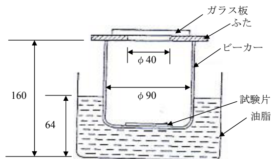
曇価試験装置
