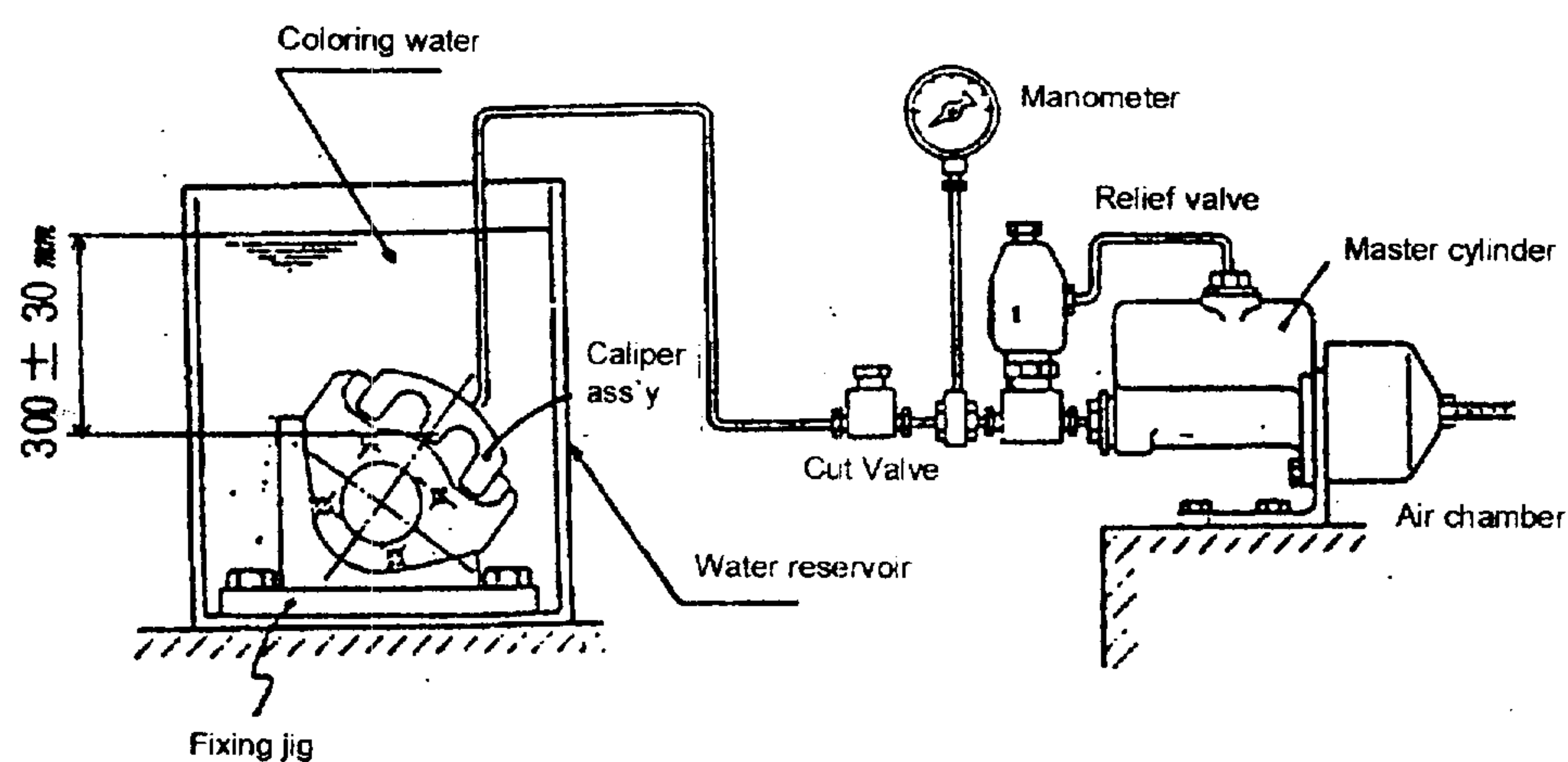
Fig. 1 Test unit
