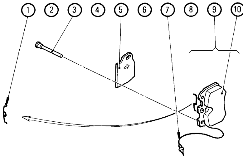
DEFINITION DES POSITIONS DES PLAQUETTES FREIN SUR LE VEHICULE
