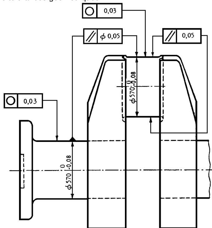
Figure 1 - Partie d'un arbre-manivelle
