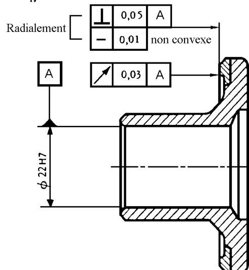
Figure 1 - Partie d'un arbre-manivelle
