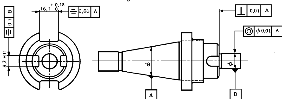
Figure 5 - Cône d'emmanchement
