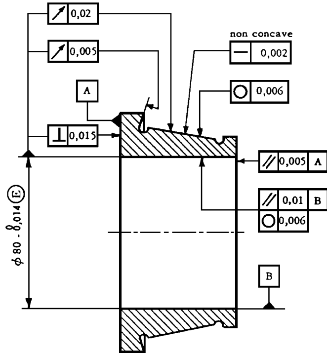
Figure 6 - Bague intérieure de roulement à rouleaux coniques
