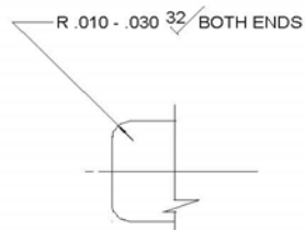
VIEW A-A
