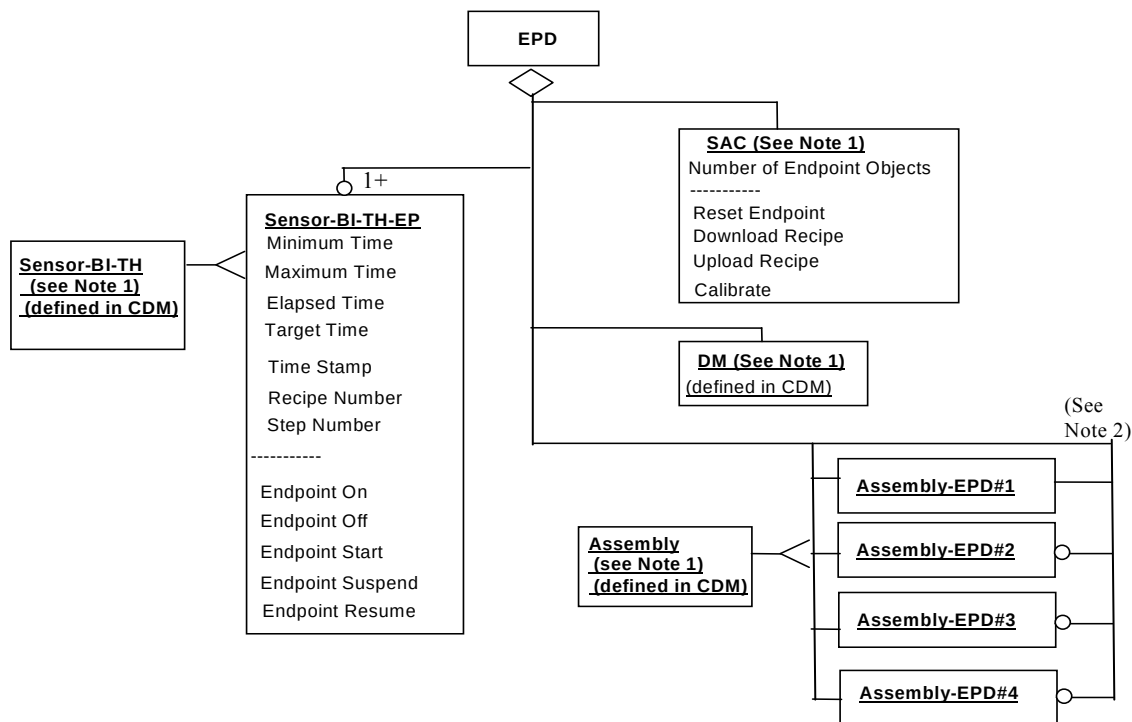
図 1 エンドポイントデバイスの高レベル構造
