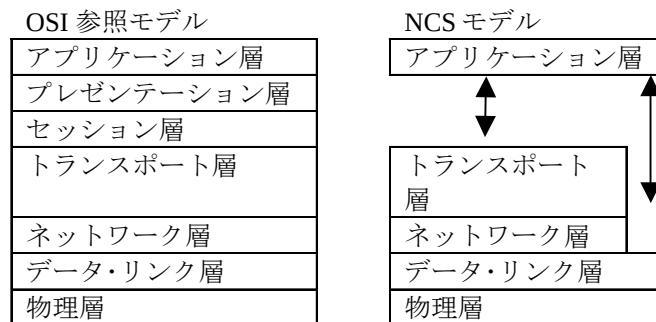
図 1 OSI に対する PROFINET の階層
