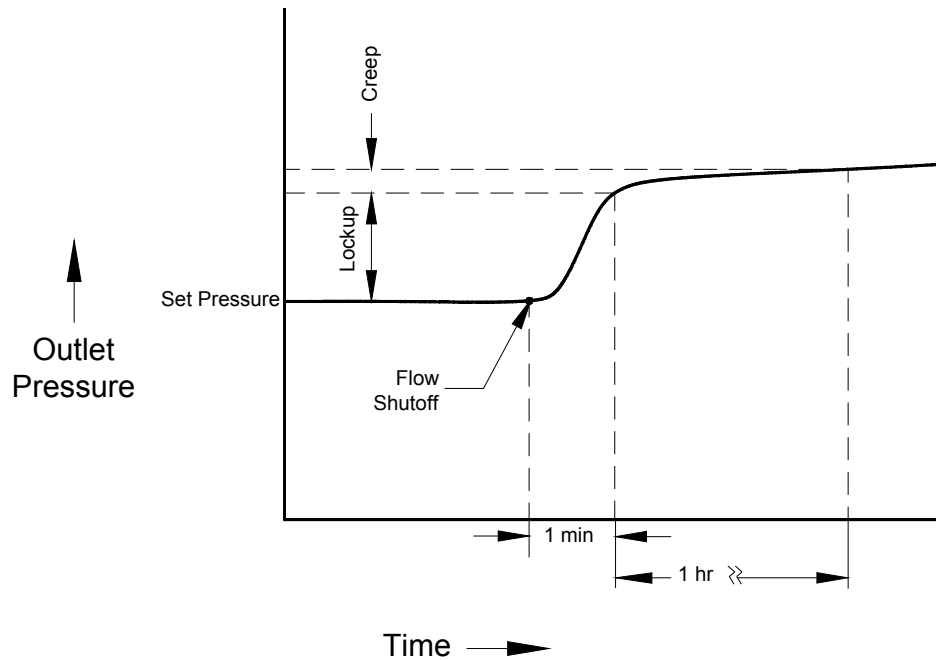
図 2 ロックアップおよびクリープ圧力
