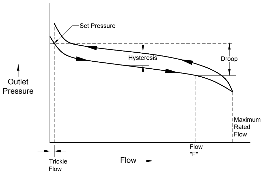
図 1 代表的な圧力レギュレータの流量曲線
