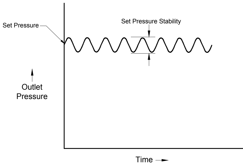
図 3 代表的なレギュレータの設定圧力安定性
