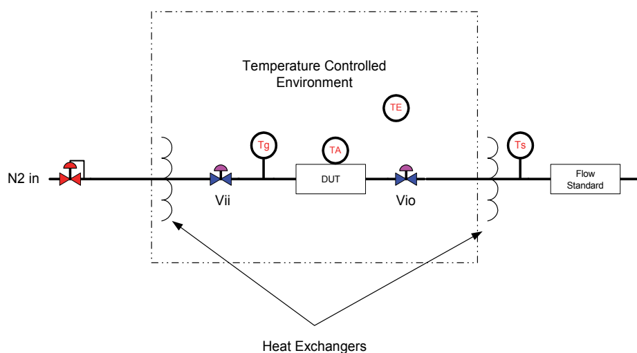
図 1 周囲温度影響の試験機器
