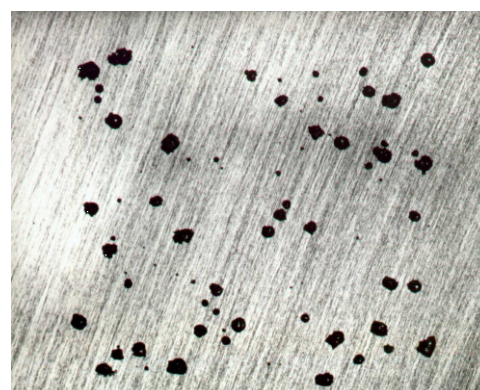
図 1 1 モルの NaCl により 25°C で実行した 孔食電位テスト後の 316 ステンレス鋼の 孔食の例 (11 倍) (17.1 項を参照)
