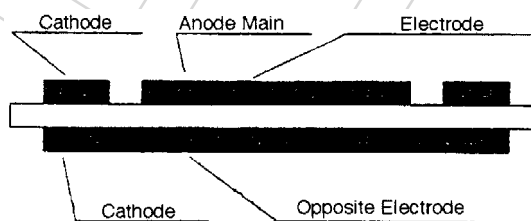
図 2B 表面抵抗率の電極接続
