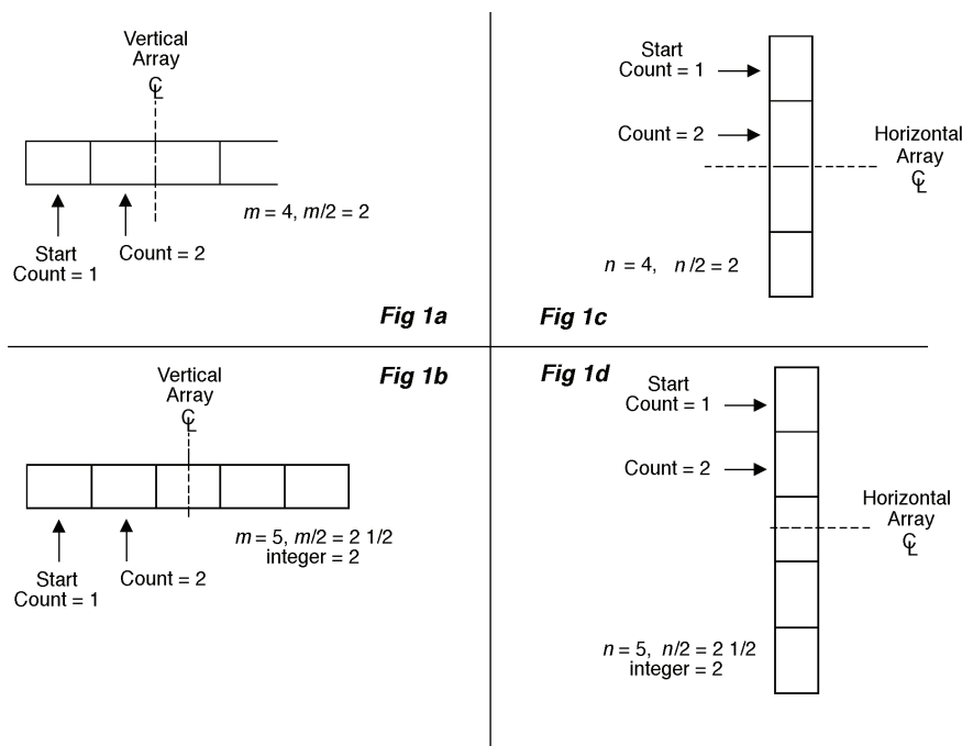
図 1 アレイセンタライン
