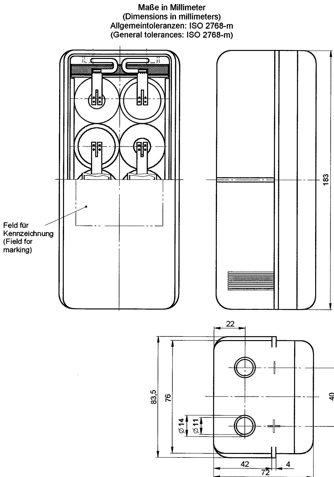
Bild 1 — Maße (Figure 1 — Dimensions)
