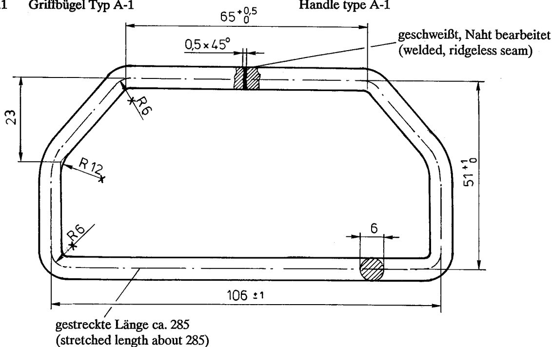
Bild 1. Griffbügel Typ A-1
