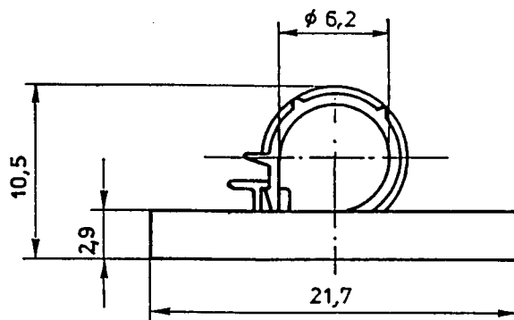
Bild 4. Klemmschelle Typ B-2
