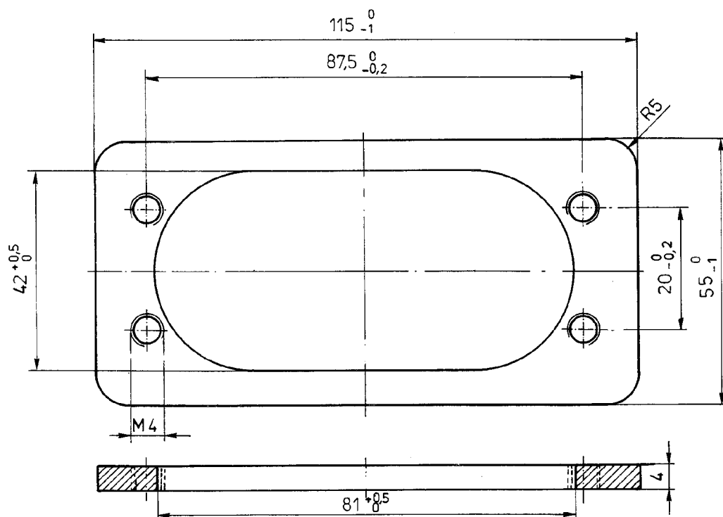
Bild 1. Befestigungsplatte
